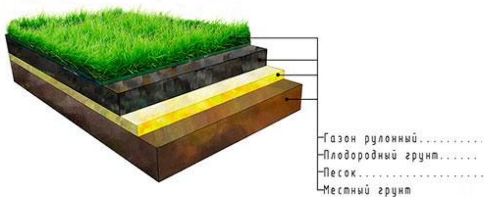
Схема устройства рулонного газона
